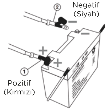
Şekil 2: Akü Montajı
