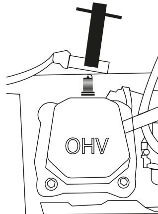
Şekil 19: Bujiyi Çıkarın
